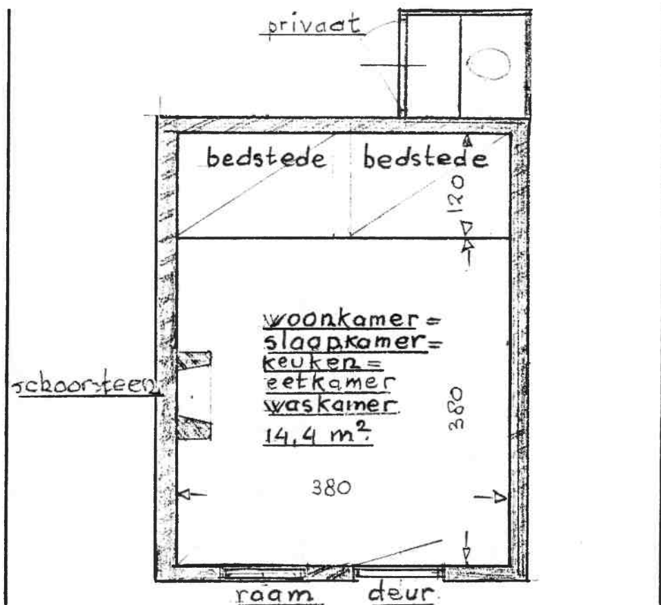
Arbeiderswoning op de Schapenkamp ( \pm 1870) Vensteroppervlak 2,2 \text{ m}^2 . Kelder: L \times B = 3,2 \times 1,8 \text{ m} . Diep: 1 \text{ m} . (tekening: Jelle Postma, 1988)
